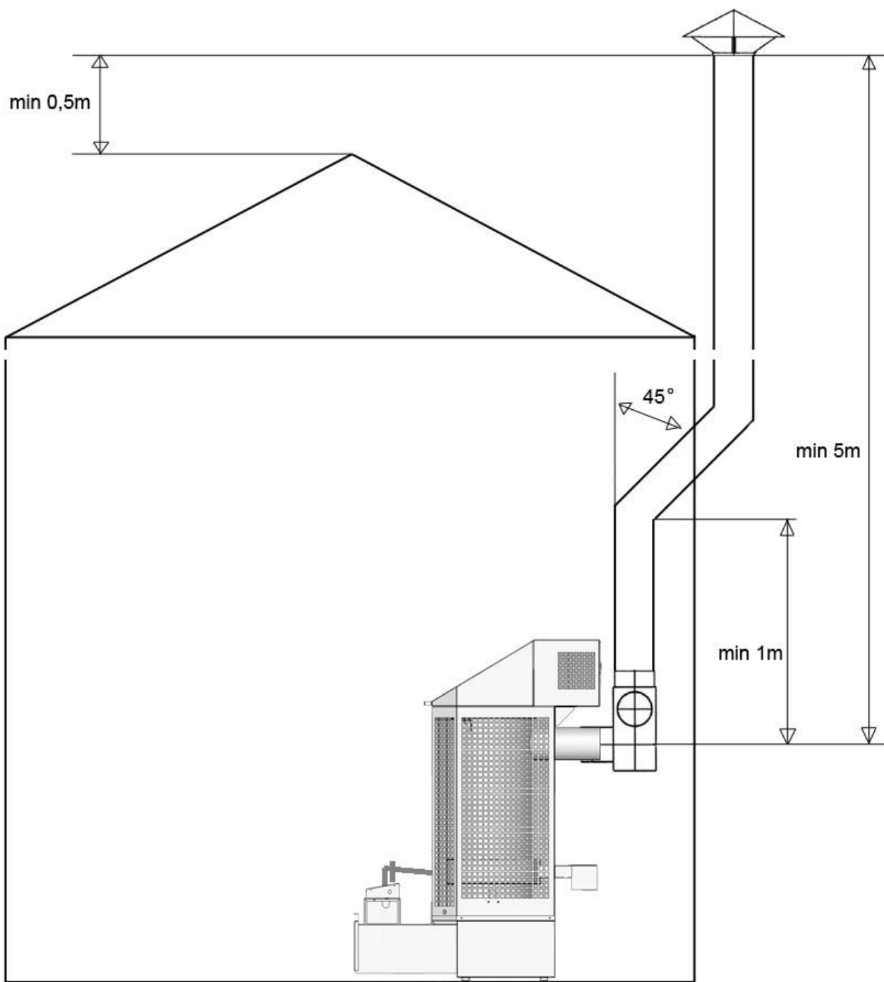
Рис. 3. Дымоходная система
