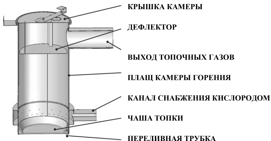
Рис. 6 Камера горения
