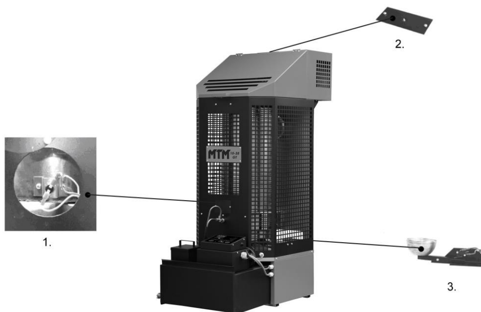
Рис. 5. Размещение предохранительных элементов нагревателя: 1. термостат возле камеры сгорания, 2. предохранение от перегрева, 3. переливное предохранение.
