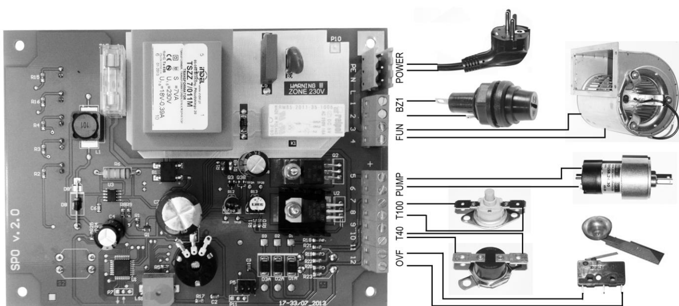
Рис. 1. Подключение контроллера нагревателя на универсальном масле, тип MTM15-35GT.
