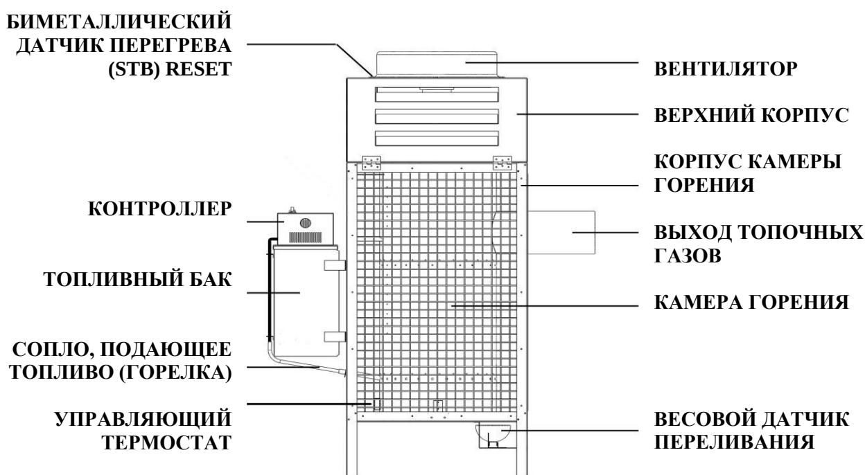
Рис. 1. Конструкция нагревателя MTM 8-30
