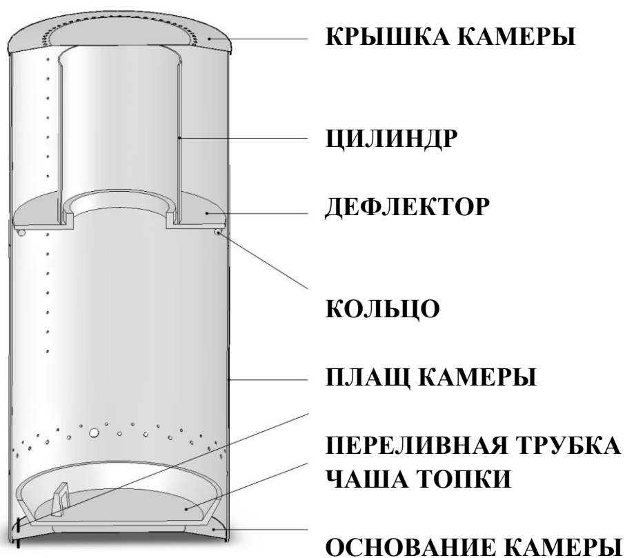
Рис. 3. Конструкция и компоненты камеры горения
