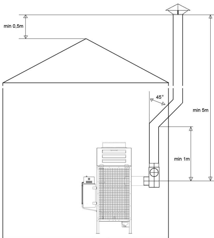
Рис. 4. Дымоходная система
