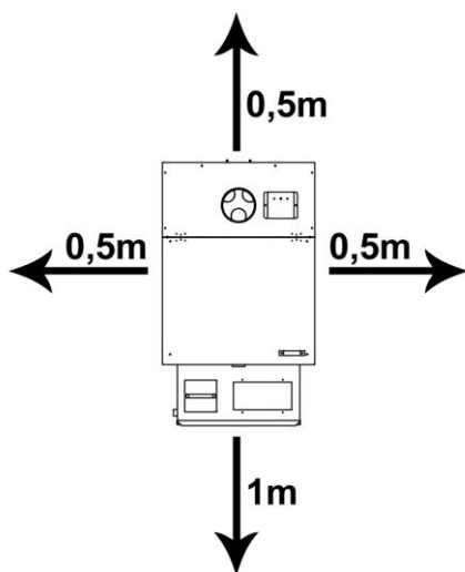
Рис. 2. Минимальное пространство безопасности вокруг устройства.
