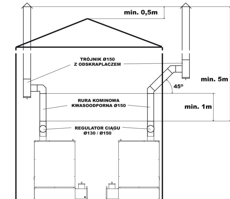
Рис. 4. Дымоходная система
