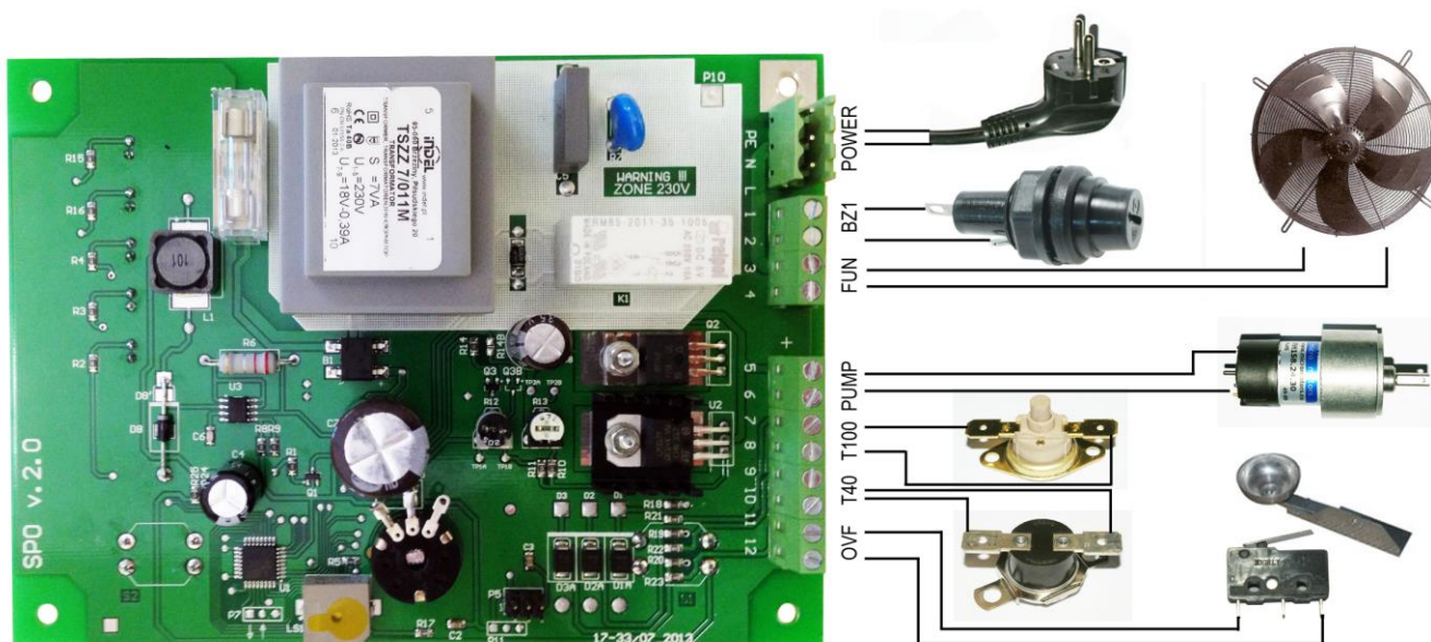
Рис. 1. Подключение контроллера нагревателя на универсальном масле, тип MTM 52.
