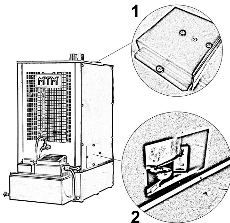
Рис. 6. Размещение предохранительных элементов нагревателя: 1. Управляющий термостат и термостат STB 2. Переливное предохранение (микровыключатель)
