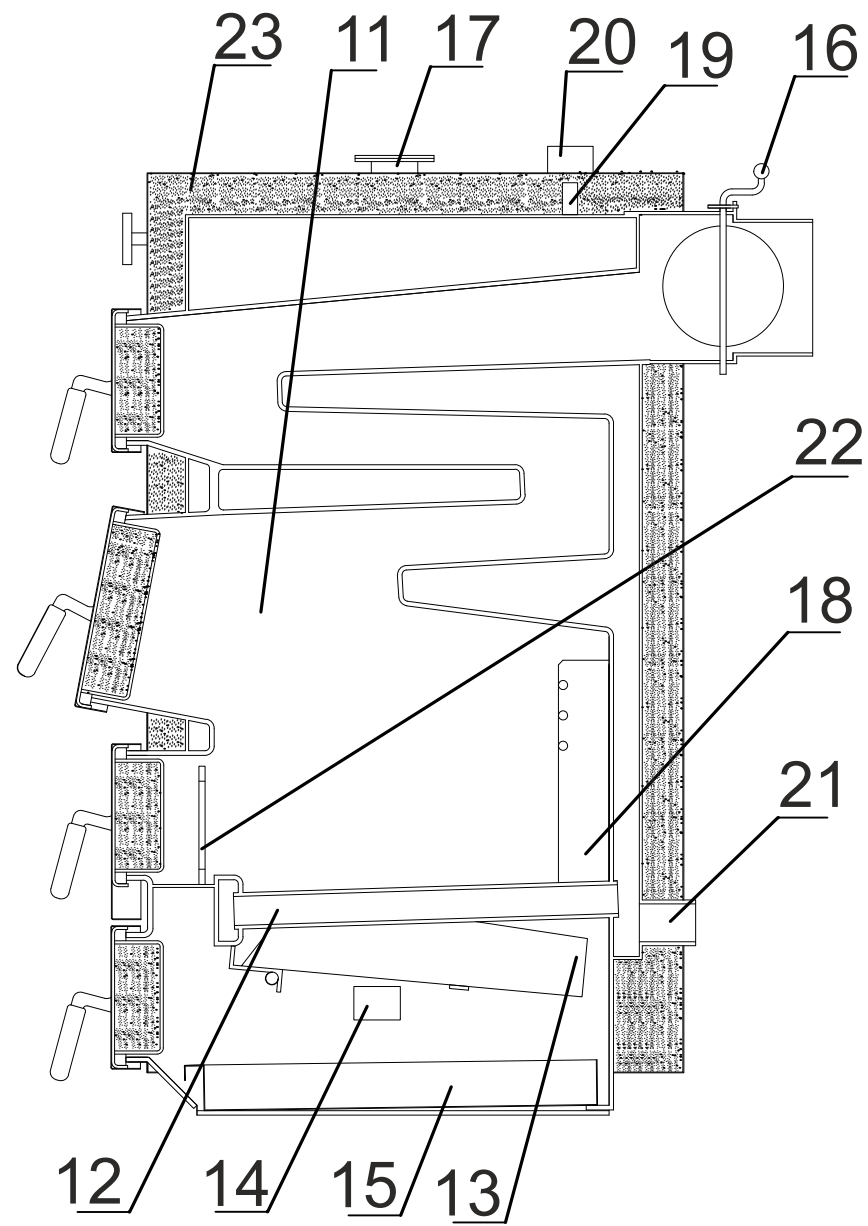
Рисунок 7.1 Основные элементы конструкции котла SE MAX II
