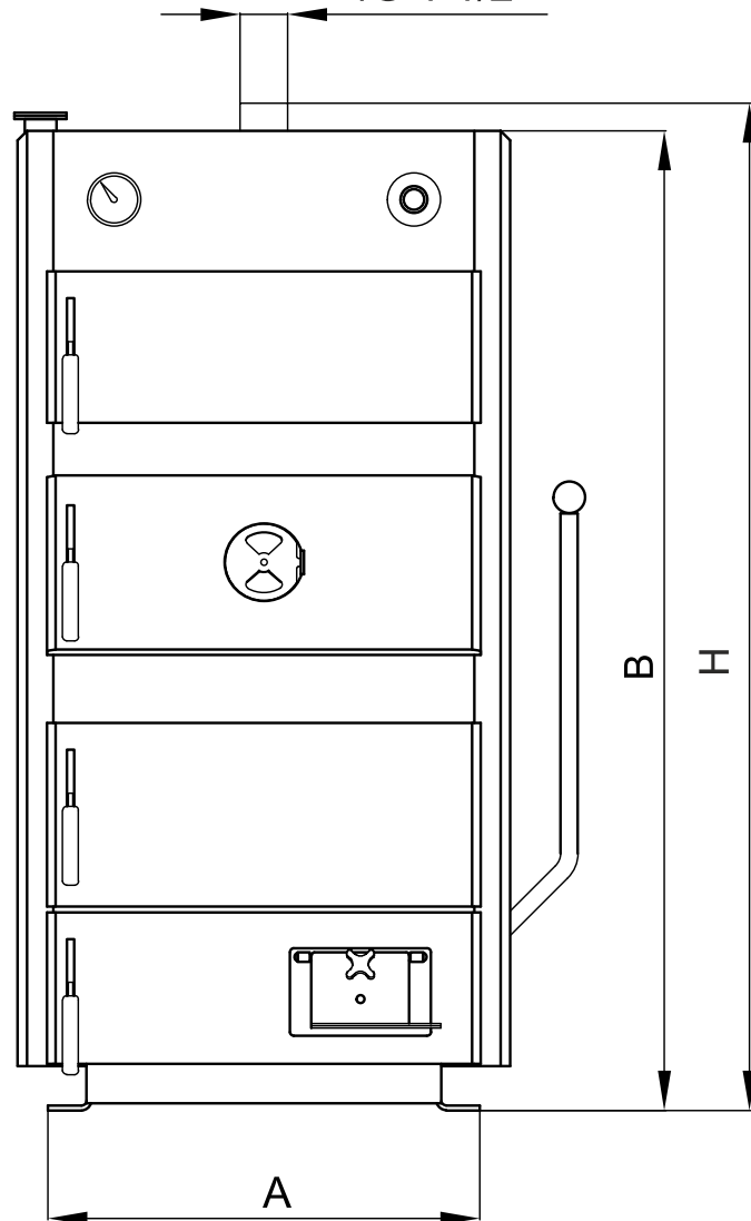
Рисунок 7.2.1 Размеры котла SE MAX II
