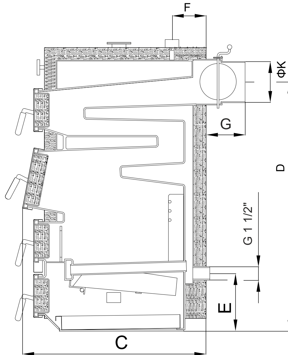
Рисунок 7.2.1 Размеры котла SE MAX II
