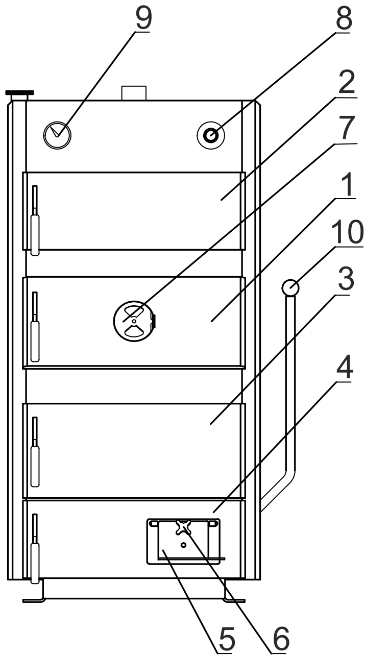
Рисунок 7.1 Основные элементы конструкции котла SE MAX II
